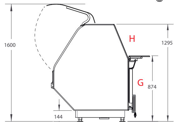
Vista Lateral
