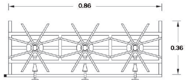
PLANTA
